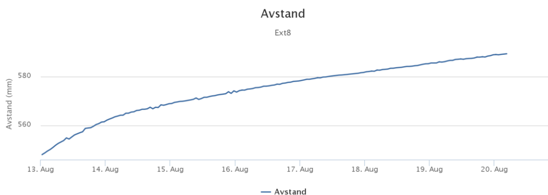
Figur 2 Bevegelsene på ekstensometer 8 den siste uka. Figur 1 viser hvor dette er plassert.
