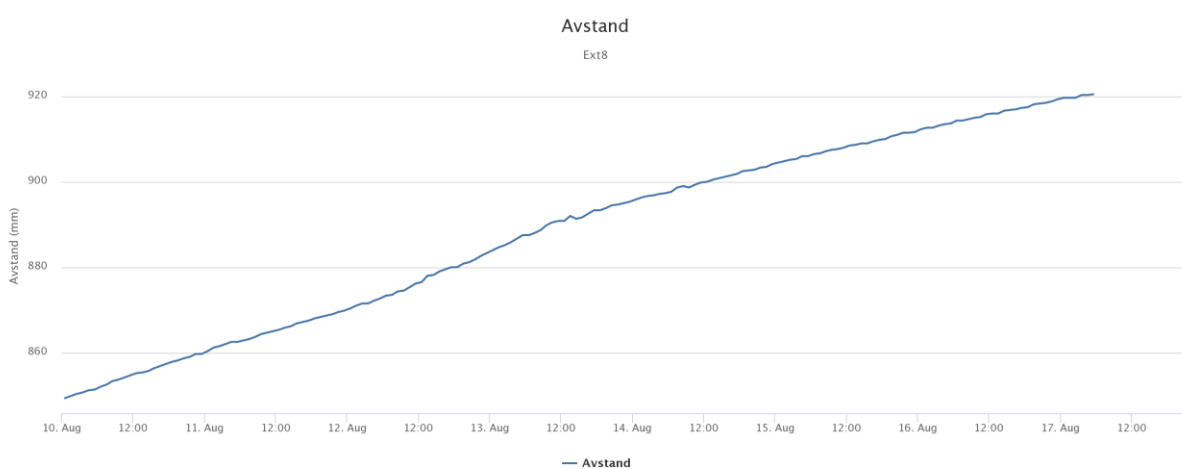
Fig. 2. Bevegelse målt på ekstensometer 8.
