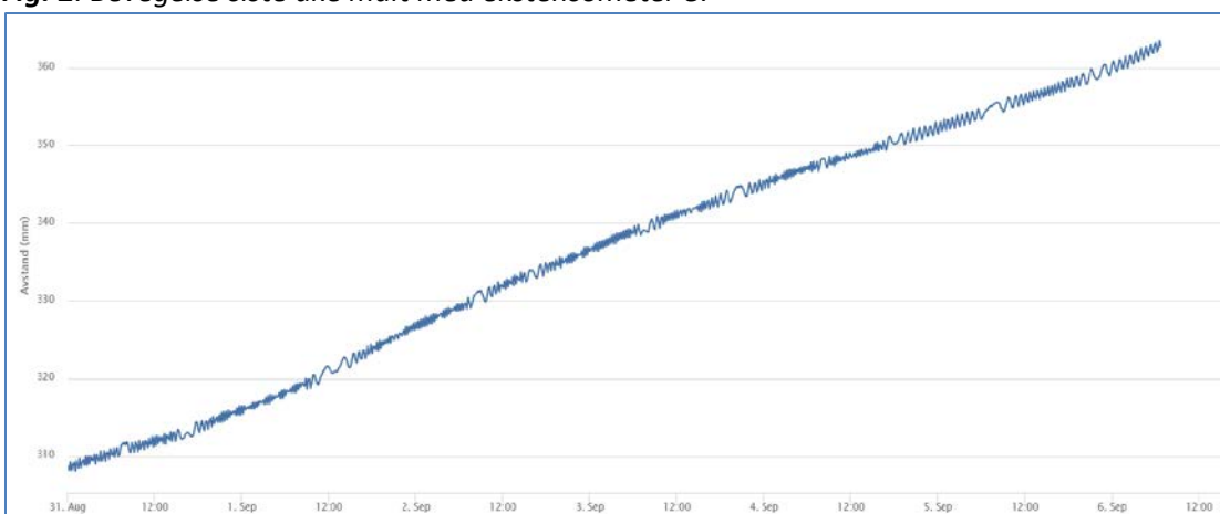
Fig. 2. Bevegelse siste uke målt med ekstensometer 8.
