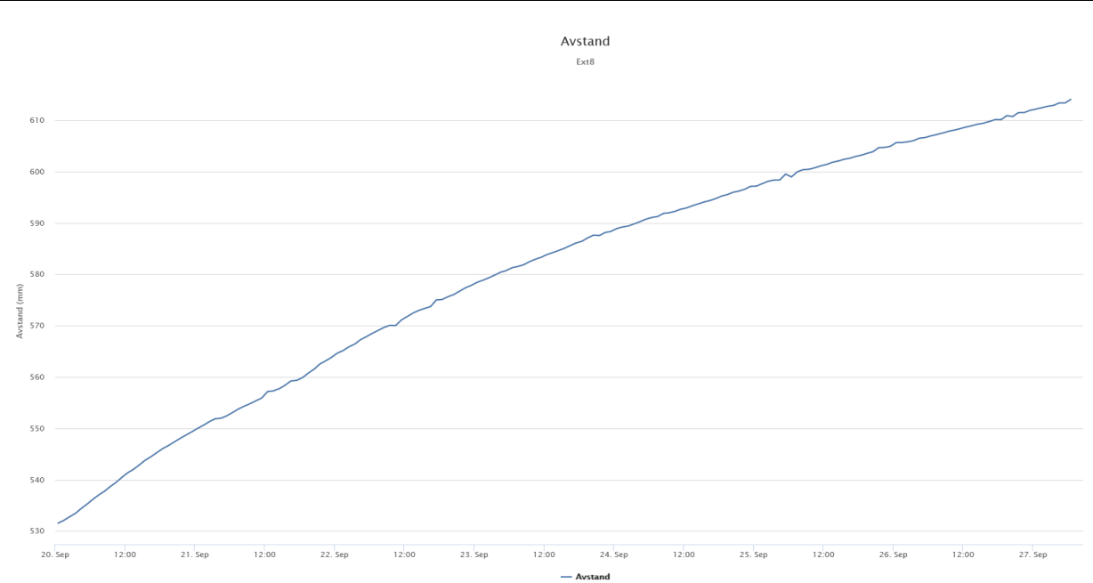
Fig. 2. Bevegelse siste uke målt med ekstensometer 8
