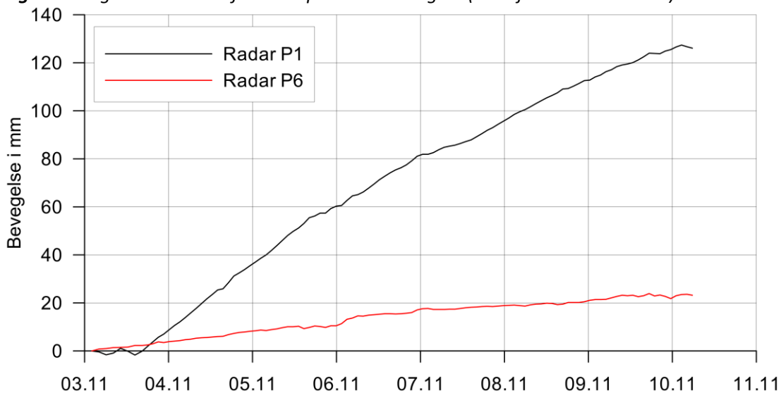
Fig. 2. Bevegelser siste uke for radarpunktene P1 og P6 (lokasjon: se kartet over)
